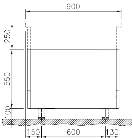
Zij aanzicht
